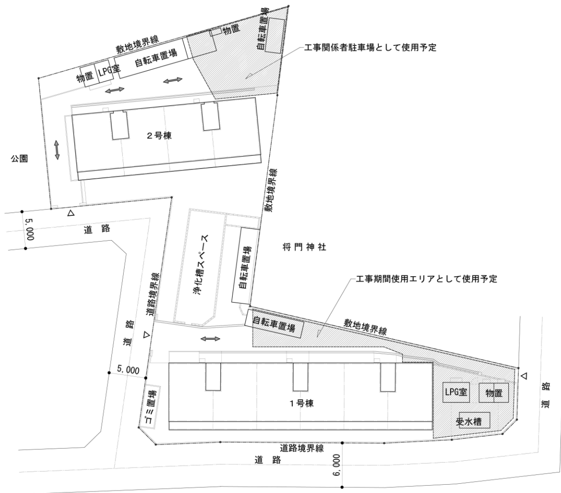
日秀団地 配置図 工事使用エリア計画
