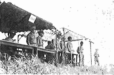
柏・我孫子合同 水防訓練おわる 七月二十九日、柏市和我孫子町の共催で連合水防訓練が柏市布佐地先の堤防でおこなわれました。当日は両市町の消防団員約五百名が参加のもとに水防の各種工法の演習をおこないました。 上・指令所 下・月の輪工法
