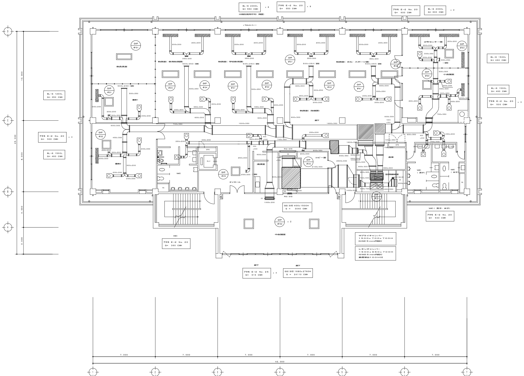
4 階 平 面 図 S=1/100
