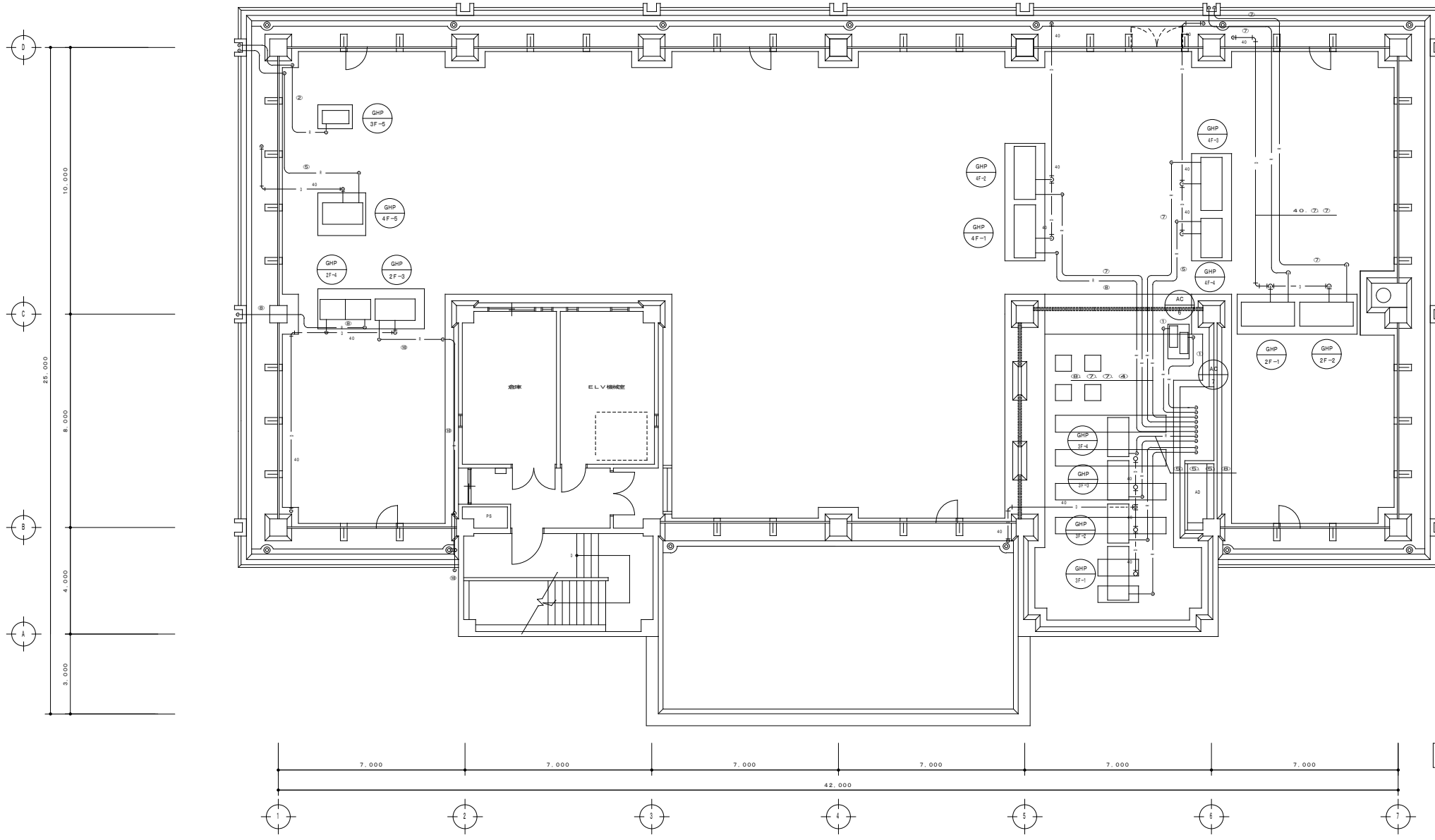
R 階 平 面 図 S=1/100
