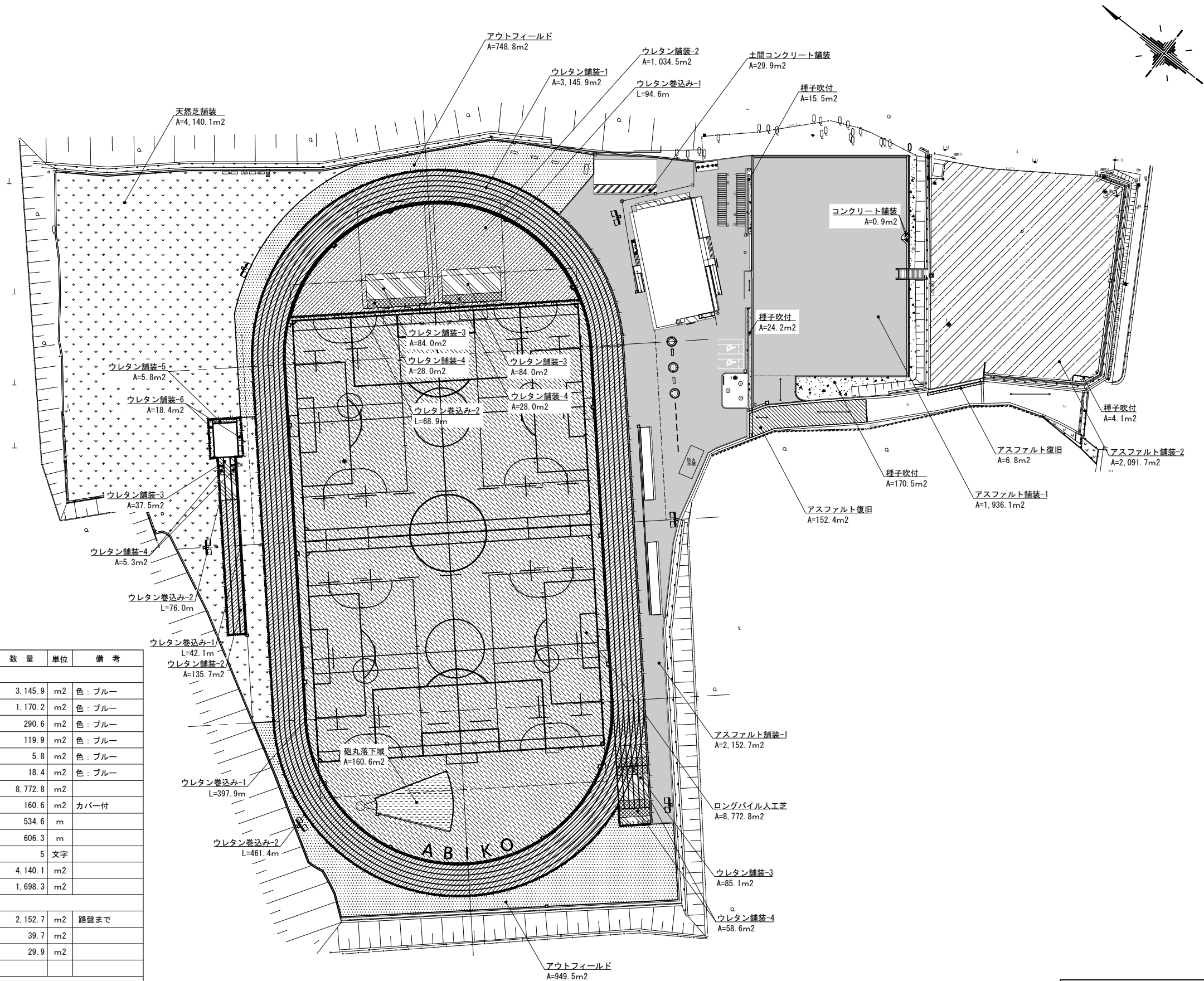
全体舗装平面図
