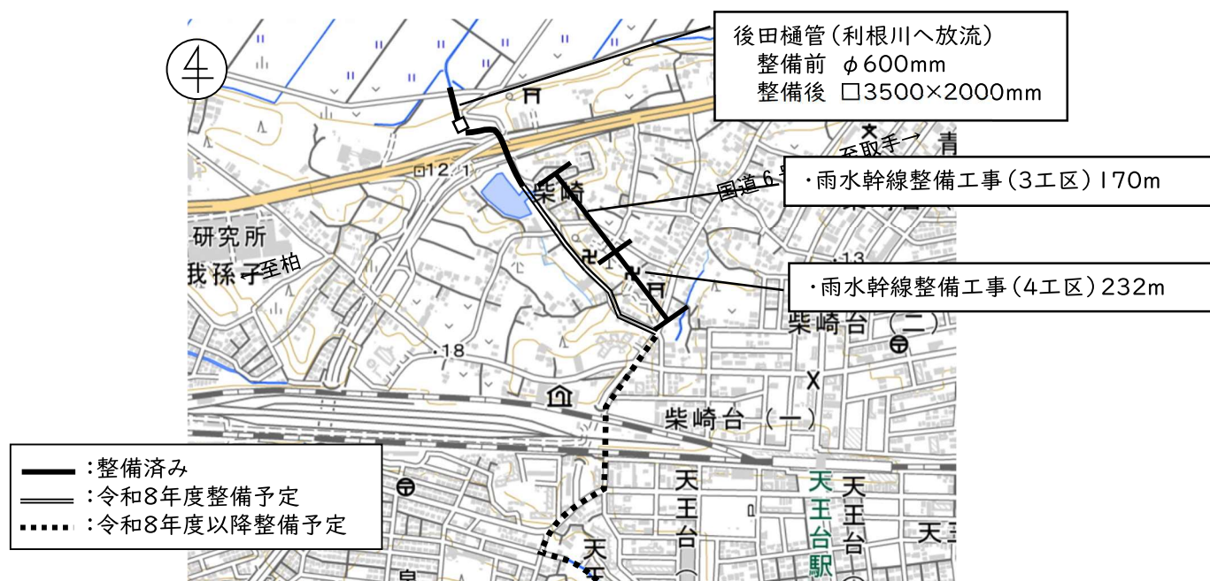
柴崎排水区整備事業の概要図
