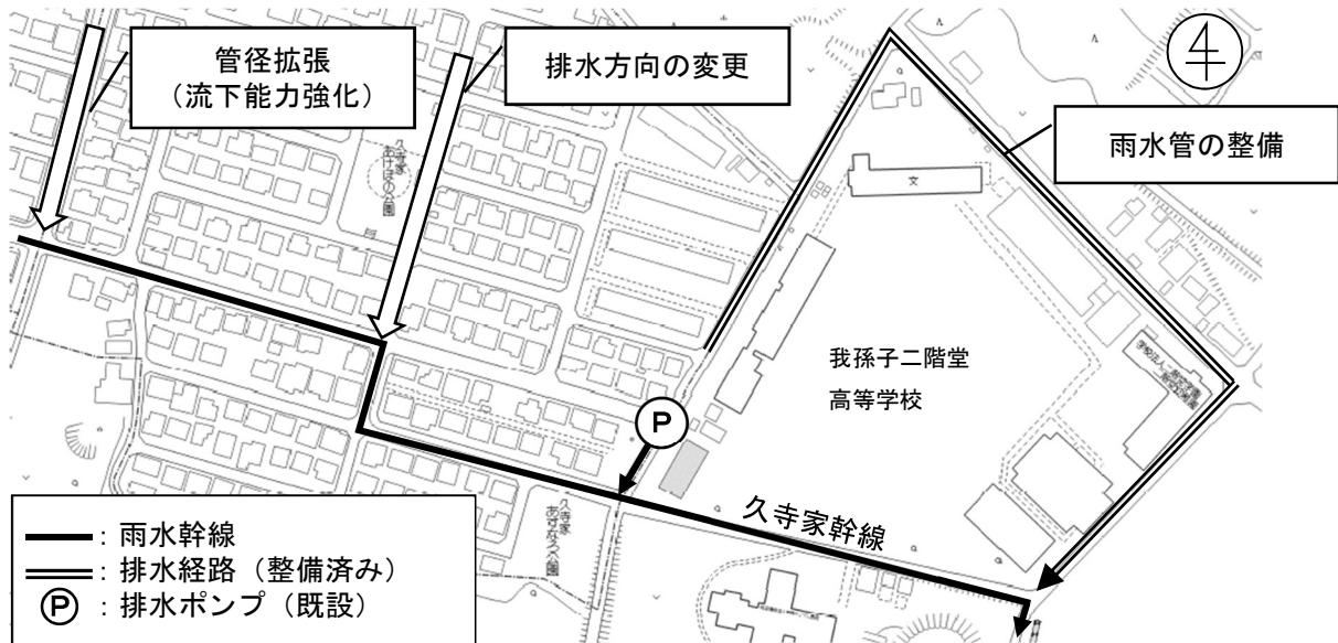
久寺家第1排水区整備事業の概要図
