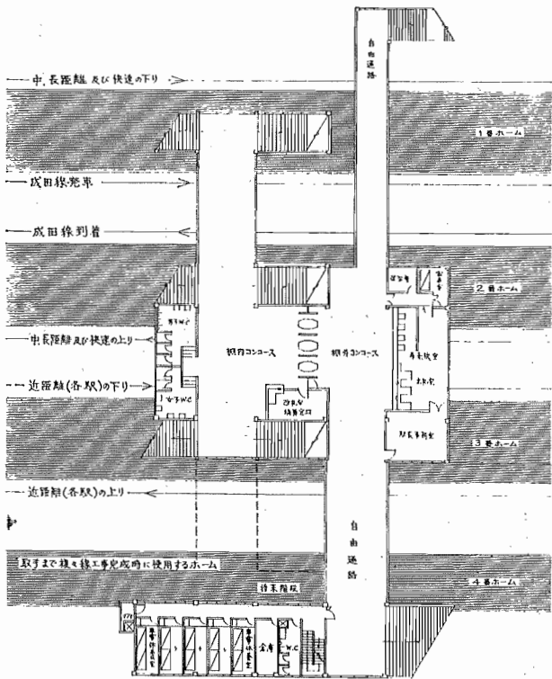
(2階平面図)
