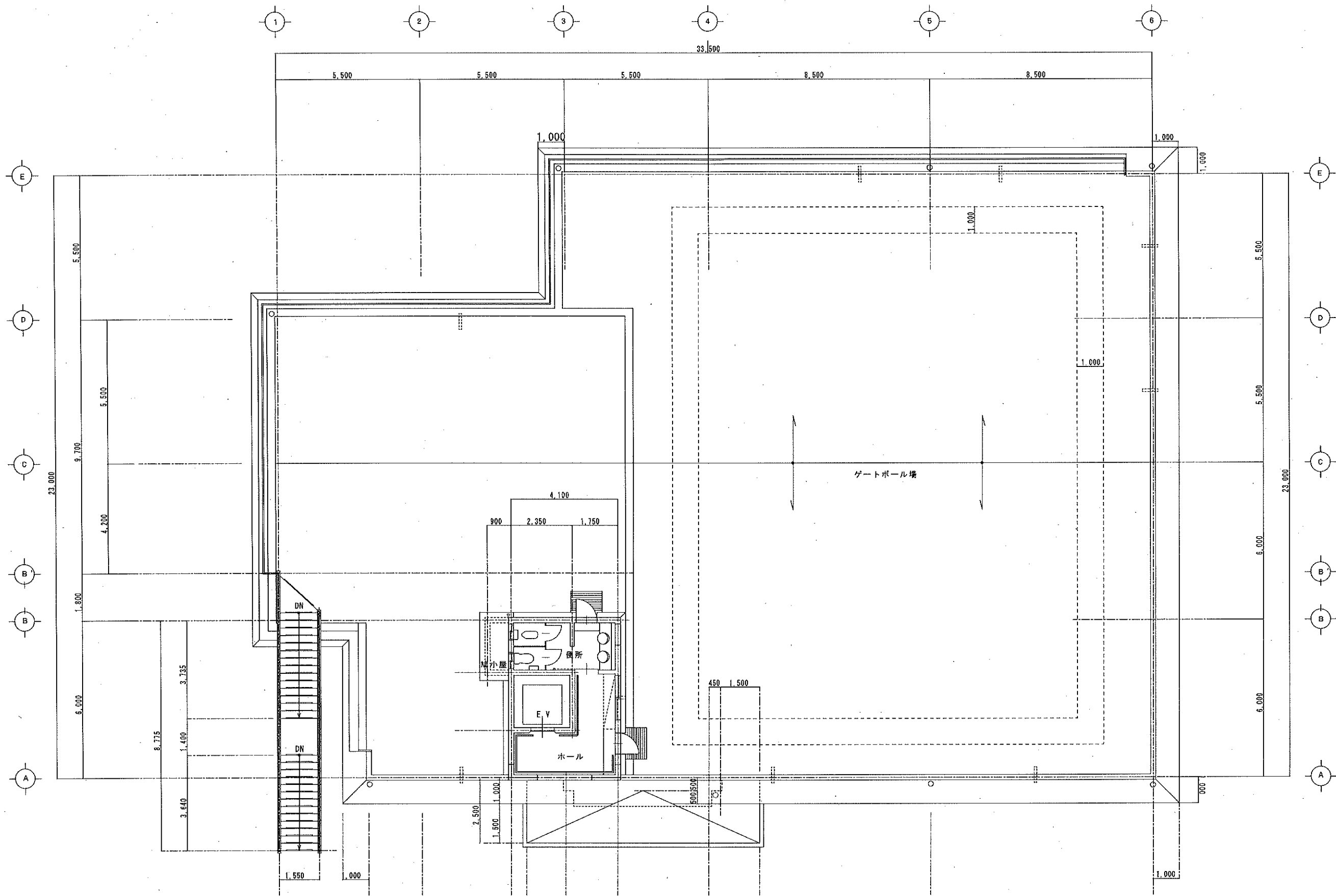
2階平面図
