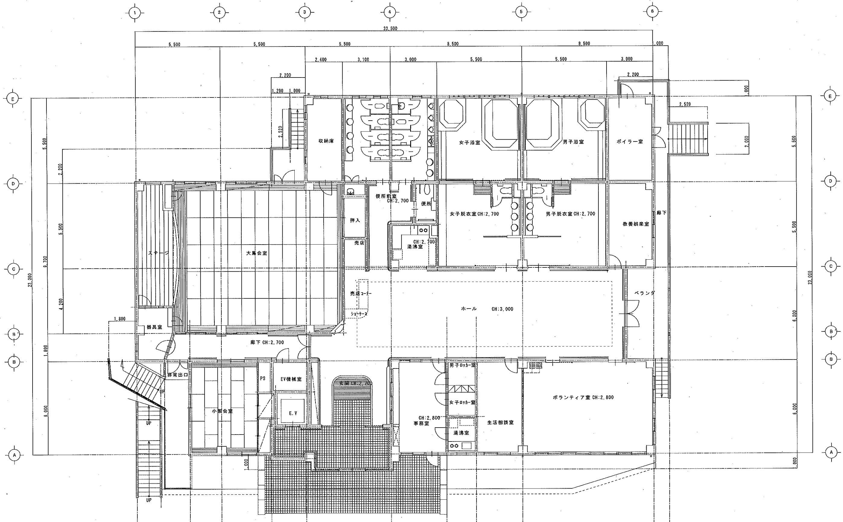
1階平面図
