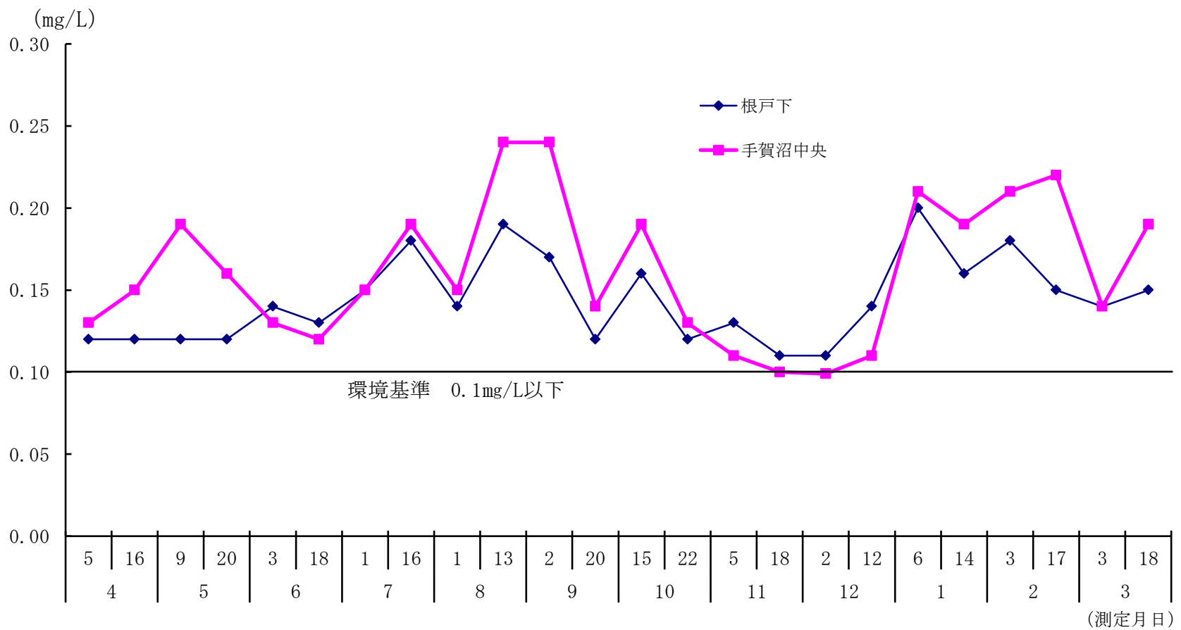
図1-10 手賀沼の全リンの月別変化 (平成25年度)
