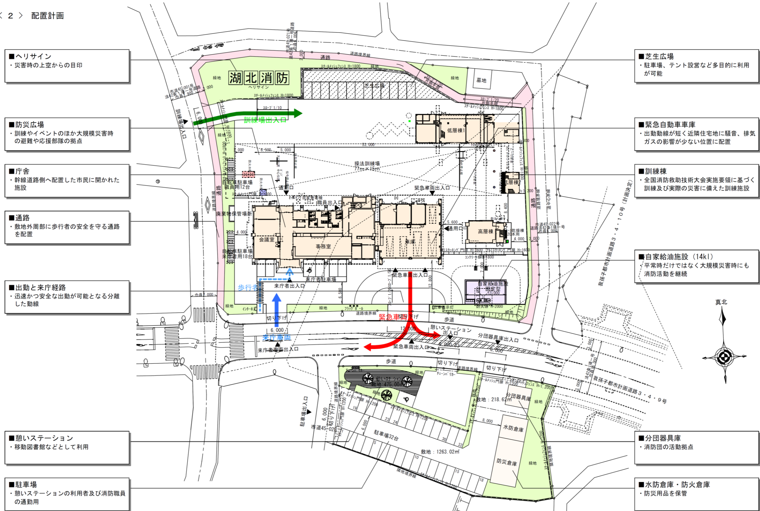
配置図 S=1/600
